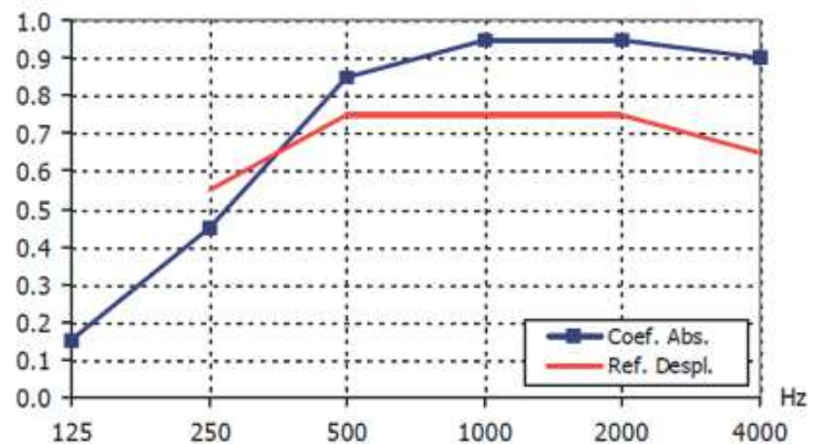
Coeficiente de absorción acústica práctico, \alpha_p
